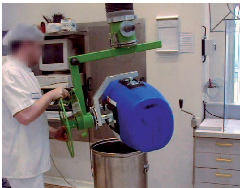
Basculeur de fût manuel.
